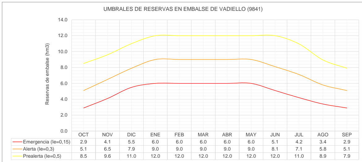
Figura 313. Umbrales mensuales para cada escenario para las reservas en embalse de Vadiello (9841) de la UTE 14 Sistema de abastecimiento de Huesca
