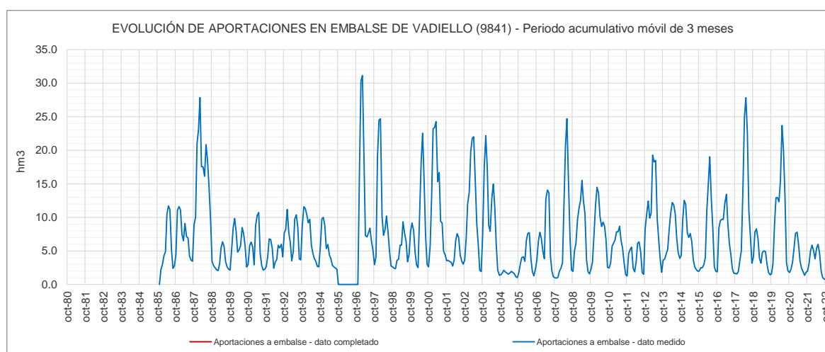
Figura 310. Evolución de las aportaciones en el embalse de Vadiello (9841) acumuladas en 3 meses de la UTS 14 Sistema de Abastecimiento de Huesca
