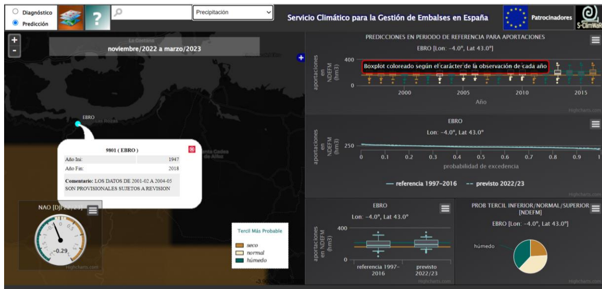
Figura 369. Predicciones del visor Web S-ClimWaReS5 en el embalse del Ebro para el periodo de noviembre 2022 a marzo de 2023.
