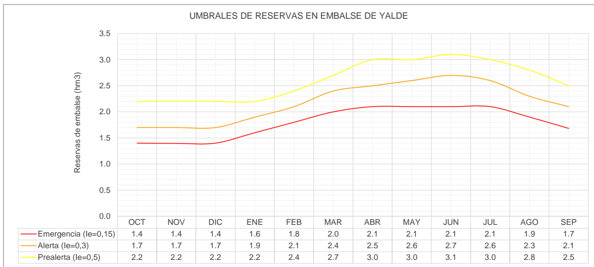
Figura 318. Umbrales mensuales para cada escenario para las reservas en embalse de Castroviejo de la UTE 03 Sistema Yalde
