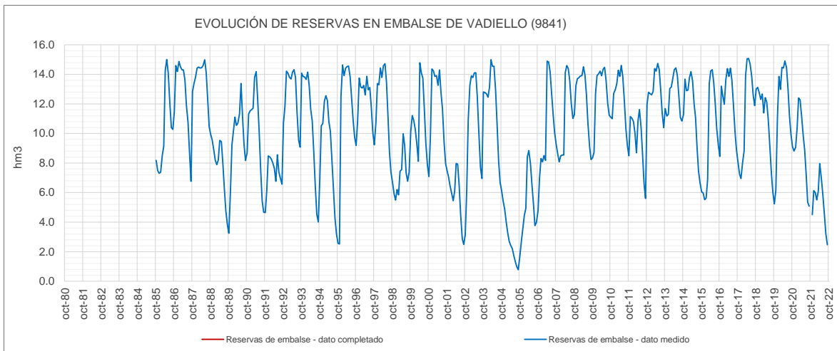
Figura 312. Evolución de las reservas en embalse de Vadiello (9841) de la UTE 14 Sistema de abastecimiento de Huesca
