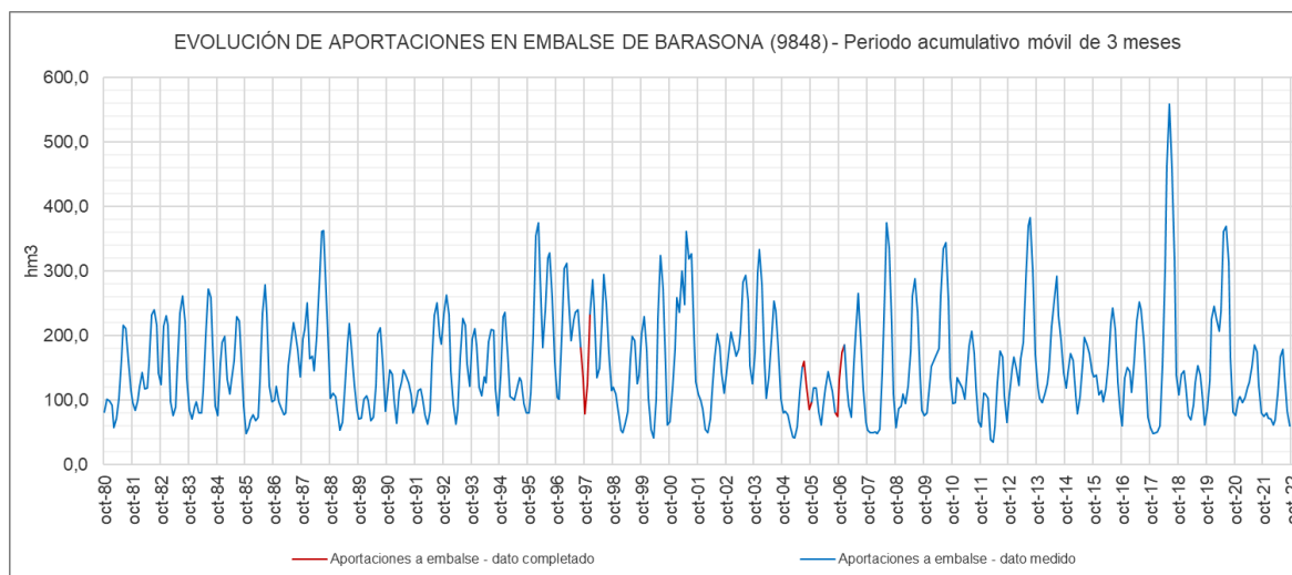
Figura 116. Evolución de las aportaciones en el embalse de Barasona (9848) acumuladas en 3 meses de la UTS 13
