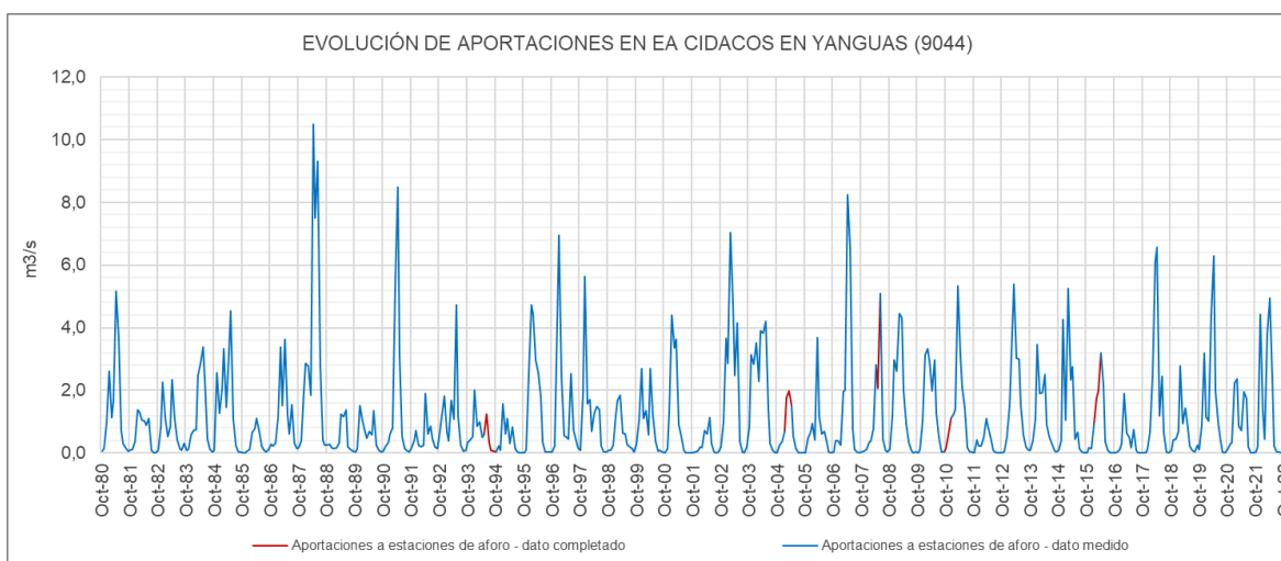
Figura 176. Evolución de las aportaciones en la estación de aforo Cidacos en Yanguas (9044) de la UTE 04
