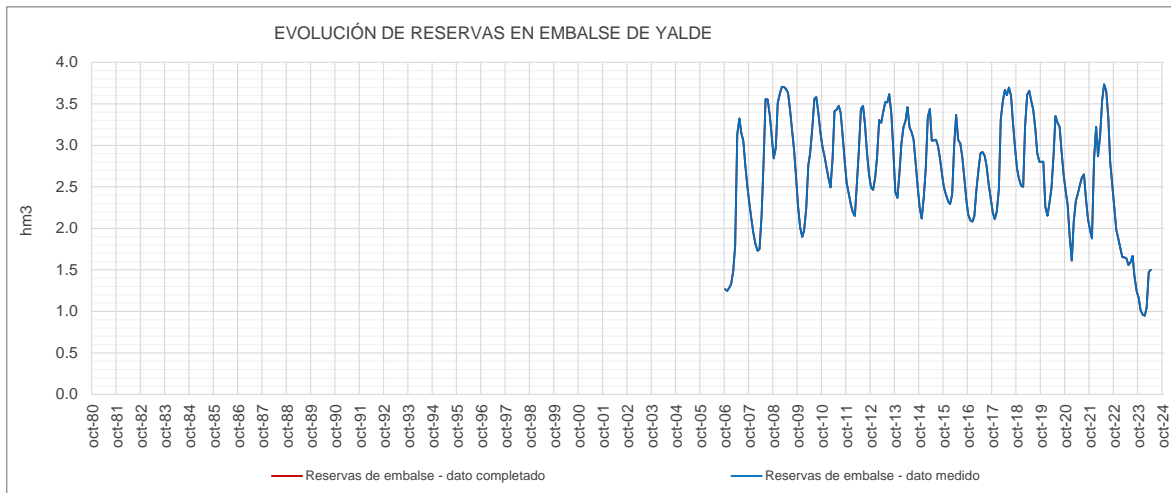
Figura 317. Evolución de las reservas en embalse de Castroviejo de la UTE 14 Sistema Yalde
