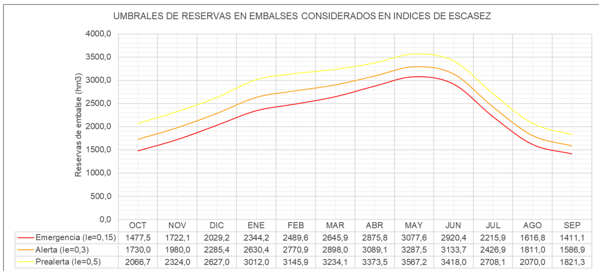
Figura 325. Umbrales resultantes para el conjunto de reservas embalsadas en todos los embalses destinados principalmente a USOS CONSUNTIVOS considerados en los indicadores de escasez, para la serie de referencia.
