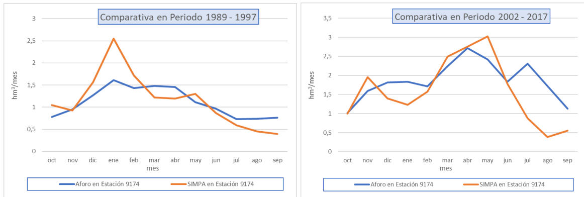
Figura 15. Comparación de la aportación media mensual de la serie registrada en la estación 9174 Río Queiles en Los Fayos con su aportación natural simulada mediante SIMPA (hm³/mes).
