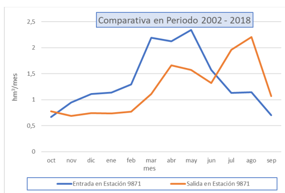
Figura 10. Comparación de la aportación media mensual entrante y saliente de 9871 Embalse Val (hm³/mes).
