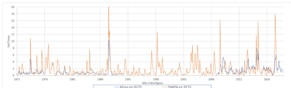
Figura 17. Comparación de la serie de aportación registrada en la estación 9175 Río Queiles en Tudela con la natural simulada mediante SIMPA (hm³/mes).
