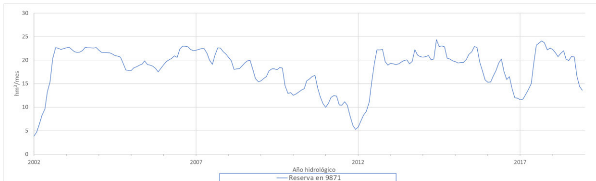
Figura 9. Almacenamiento registrado en 9871 Embalse Val (hm³/mes).
