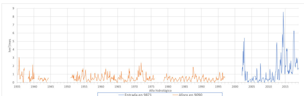
Figura 11. Comparación de la serie de aportación entrante en 9871 Embalse Val con la registrada en la estación 9090 Barranco Val en Los Fayos (hm³/mes).
