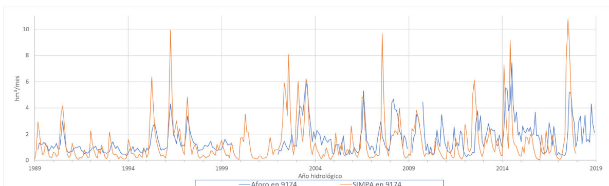
Figura 14. Comparación de la serie de aportación registrada en la estación 9174 Río Queiles en Los Fayos con la natural simulada mediante SIMPA ( \text{hm}^3/\text{mes} ).
