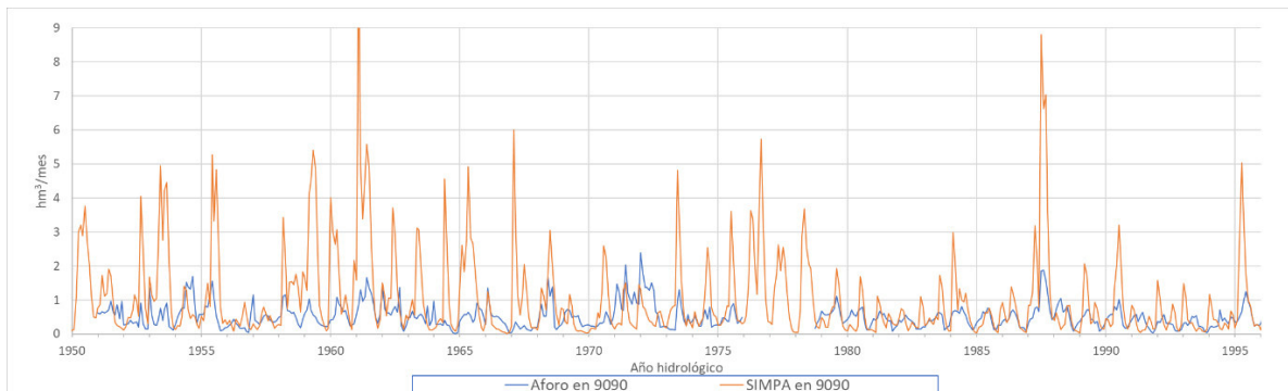
Figura 12. Comparación de la serie de aportación registrada en la estación 9090 Barranco Val en Los Fayos con la natural simulada mediante SIMPA ( \text{hm}^3/\text{mes} ).
