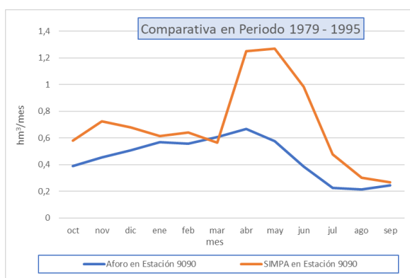
Figura 13. Comparación de la aportación media mensual de la serie registrada en la estación 9090 Barranco Val en Los Fayos con su aportación natural simulada mediante SIMPA ( \text{hm}^3/\text{mes} ).
